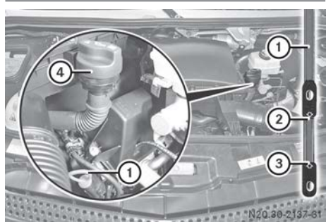
4-Zylinder Dieselmotor (Beispiel)
