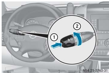
Kombischalter
