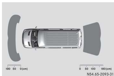
Warnanzeige Frontzone
