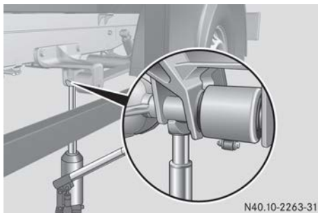
Wagenheber-Aufnahmepunkt, Hinterachse (Beispiel Pritschenfahrzeug bis 3,5 t)
