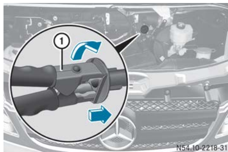
Fremdstartstützpunkt an der Stirnwand (Beispiel 4-Zylinder Benzinmotor)
