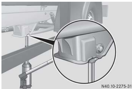
Wagenheber-Aufnahmepunkt, Hinterachse (Beispiel Pritschenfahrzeug 5 t)
