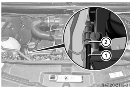
6-Zylinder-Motor
