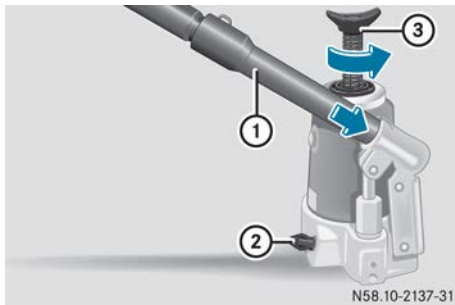
Hydraulischer Wagenheber
