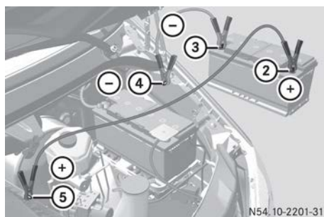
Anschlussplan (Beispiel)
