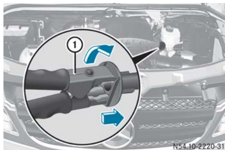
Fremdstartstützpunkt links am Luftfilter (Beispiel 6-Zylinder Motor)
